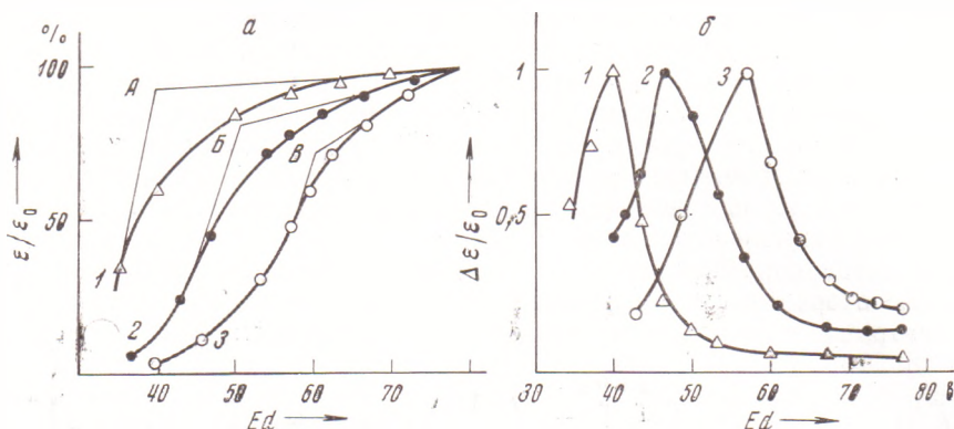
Рис. 2. a — зависимость относительной эффективности к.э.у. от ускоряющего потенциала в сечении канала при облучении электронами (1), протонами (2) и ультрафиолетовым излучением (3); б — результат дифференцирования зависимостей \varepsilon/\varepsilon_0 = f(Ed)
