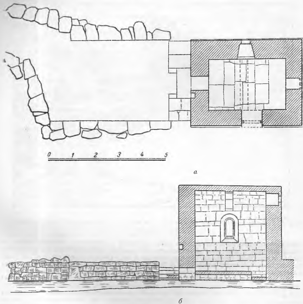
Рис. 2. Голианкская церковь (по материалам Триалетской этнографической экспедиции): а — план; б — разрез
