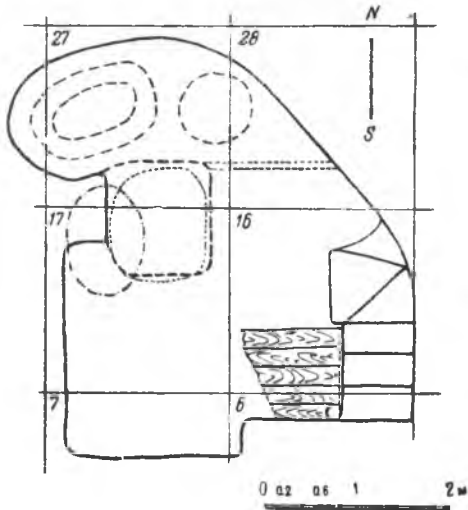
Рис. 1. План полуземлянки
