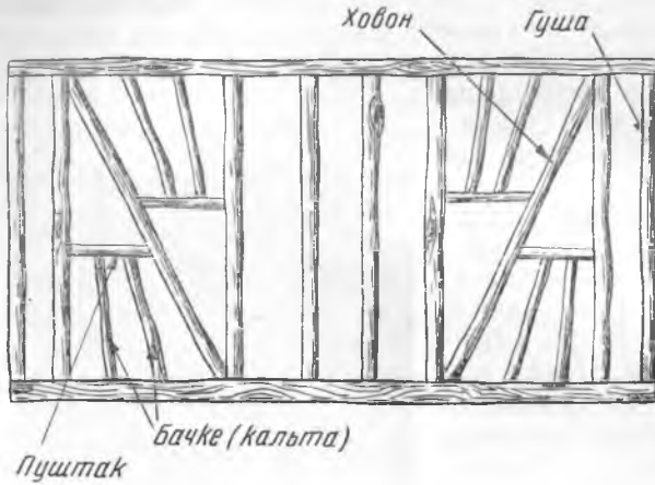
Рис. 2. Система каркаса
