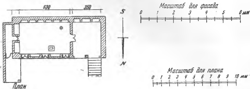
Рис. 14. Дом XIX в. в Шахрисябзе. Жилая комната с айваном. Позади примыкает мадан. Обмер автора. Ин-т искусствознания УзССР
