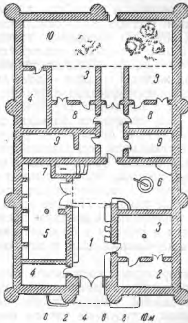
Рис. 19. Сельская усадьба хаули в сел. Пышканик близ Хивы. а — фасад, б — план: 1 — долон; 2 — михманхона; 3 — айван; 4 — кавчок; 5 — атхона; 6 — хараз; 7 — бадраб; 8 — уй; 9 — пеш уй; 10 — саан. Обмер автора. Ин-т искусствознания УЗССР
