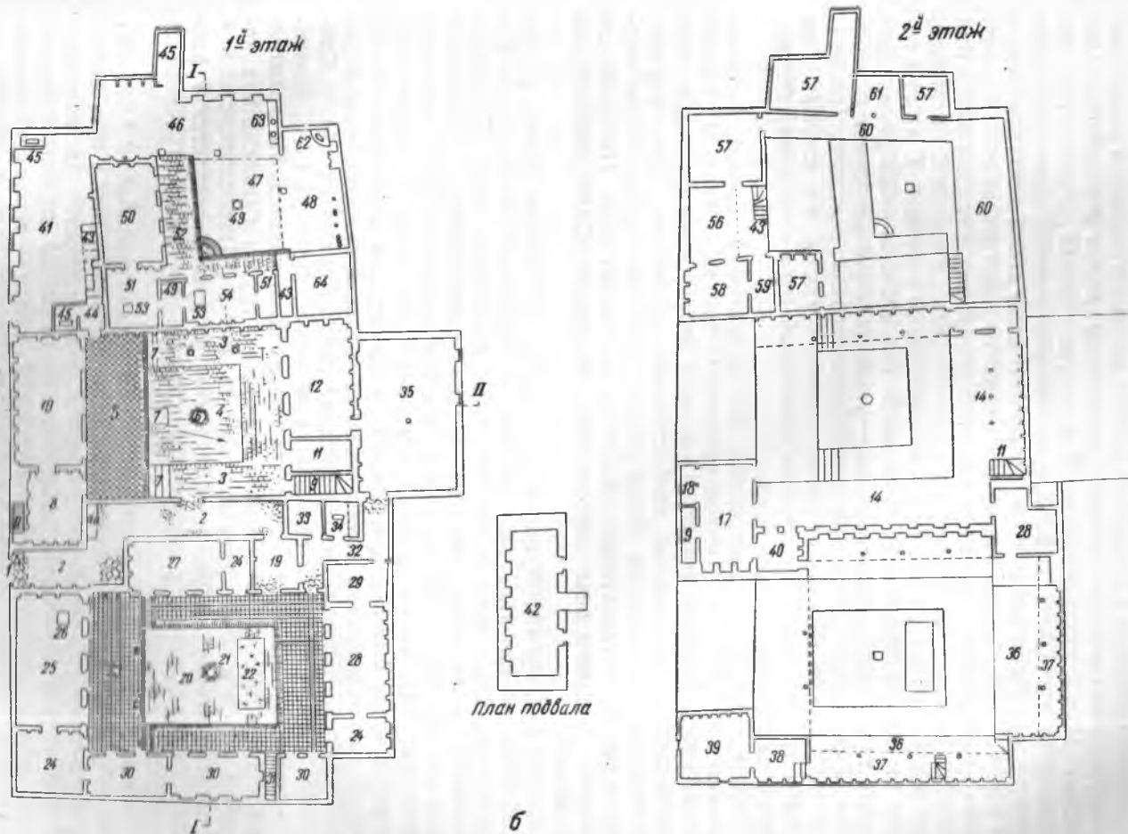
Рис. 13. Дом купца Мирзо Хабиб Хурдова в Бухаре; а — разрез; б — план, Бирун: 1 — дарназа; 2 — рахрау; 3 — руи-хаули (открытый двор); 4 — суфа; 4а — суфача; 5 — летняя суфа; 6 — тошнау; 7 — ступени; 8, 11 — дахлиз; 9 — зина; 10 — михмахона; 12 — хона хаули (зимняя приемная); 13 — зимняя терраса; 14 — зимний нимайзончи; 15 — зимняя болохона; 16 — летняя терраса; 17 — летняя болохона; 18 — курпа хона (для одежды); 42 — тагхона (подвал), Дарун: 19, 32 — рахрау; 20 — руи-хаули; 21 — тошнау; 22 — цегник; 23 — летний айван; 24 — дахлиз; 25 — хона-и руй-бо боле (летняя); 26 — сандал; 27 — хона-и руй-бо офтоб (комната на восток); 28 — хона-и руй-бо пойон (зимняя); 29 — мадон; 30 — хона-и руй-бо кибля (комната на запад); 31 — зина; 33 — хона (кладовая); 34 — бадраб; 35 — ашхона; 36, 37 — зимняя терраса и нимайзончи; 38 — шабга (ночная терраса); 39, 40 — летняя и зимняя болохона. Хозяйственный двор: 41 — сейсхона; 43 — зина; 44 — рахрау; 45 — бадраб; 46 — айван охур (с кормушками); 47 — руи хаули; 48 — айван; 49 — тошнау; 50, 51, 52 — хона-и руй-бо боле с передней и суфой; 53 — сандал; 54 — хона-и руй-бо кибля; 55 — мадон; 56 — летняя терраса; 57 — болохона; 58, 59 — микманхона и дахлиз; 60, 61 — терраса и нимайзончи; 62, 63 — танур и оташдон; 64 — кладовая. Обмер Тимофеева, Отдел охраны памятников при Совете Министров УзССР
