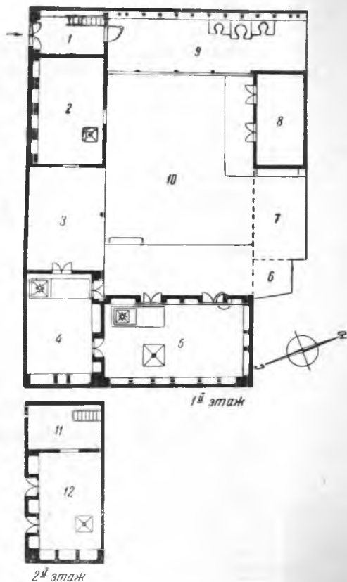
Рис. 12. Дом в квартале Козы Абдурасуль в Самарканде: 1 — дарваза-хона; 2, 4, 8 — хона; 3, 9 — айван; 5 — сеихона; 6 — бадраб; 7 — ашхона (разрушена); 10 — руихаули (двор); 11 — дахлиз; 12 — болохона. Обмер С. Н. Полупанова. Музей искусств УзССР
