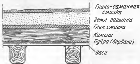
Рис. 9. Конструкция кровли
