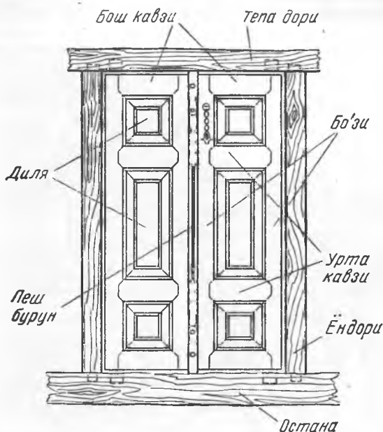
Рис. 8. Конструкция дверей
