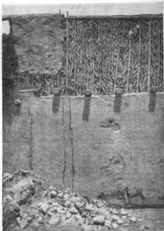
Рис. 1. Каркасная конструкция стены (Хива). Фото Музея искусств УзССР
