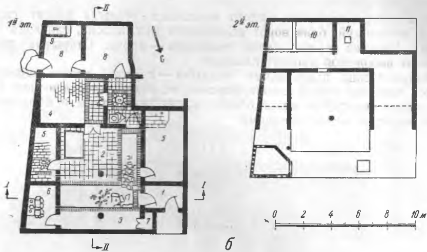
Рис. 16, б Дом XIX в. в Хиве: а — разрез, б — план: 1 — дахлиз; 2 — онг-айван; 3 — терс-айван; 4 — сарай; 5 — ямбаши-уй; 6 — ашхона; 7 — кумырхона; 8 — малхона; 9 — бадраб; 10 — таляк; 11 — световой колодезь. Обмер автора, Ин-т искусствознания УзССР
