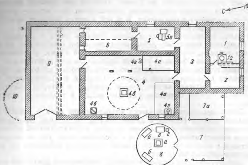
Рис. 10. План усадьбы Бекбая Утинязова, председателя колхоза им. Ахунбабаева: 1—2— зимние жилые комнаты (ожре) с печью (1а) и дощатым полом; 3— коридор-сени (дализ); 4— зимнее помещение для юрты (уйжай); а— глинобитные возвышения «суфа», накрытые циновками и кошками; б— мельница (лигирман) с ручными жерновами; в— место, где устанавливается на зиму юрта; г— очаги для варки пищи; 5— кладовая с печью (5а) для мелкой хозяйственной утвари; б— кладовая с деревянным настилом вдоль всей стены для хранения зерна и других запасов; 7— навес (шертек) возле дома с большой суфой (7а); 8— юрта; а— очаг; б— шкафчики (сантык) для посуды с уложенными сверху одеялами и подушками; в— стол; г— стул; 9— хлев (сенсхона); 10— загон для мелкого скота, сделанный из палок и ветвей (корá)
