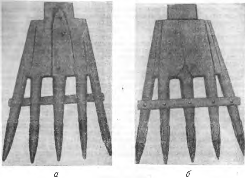
Рис. 1. «Плотина» — основная рабочая часть пятизубой сохи: а — вид спереди; б — вид сзади. Дер. Пулово-Борисово, Ирдомашского сельсовета, Череповецкого района, Вологодской обл.
