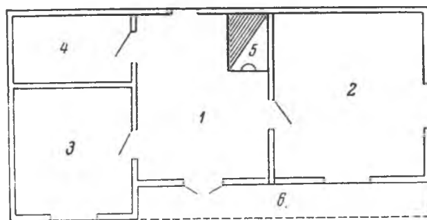
Рис. 7а. План новой хыжи в Воловом. 1—кухня, 2—«велика хижа». 3—«мала хижа», 4—комора, 5—плита, 6—ганок (масштаб: в 1 см 1 м)
