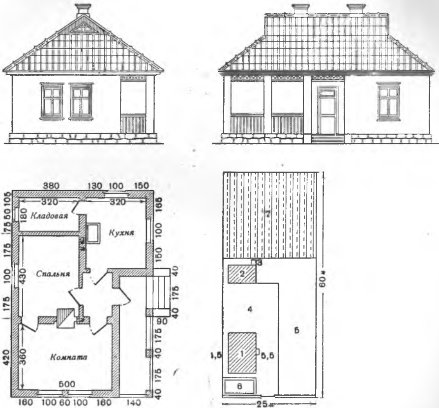
Рис. 5. План и внешний вид дома в селе Вилко. Постройка 1948—1949 гг. 1—жилой дом, 2—сарай, 3—уборная, 4—хоз. двор, 5—сад, 6—цветник, 7—огород
