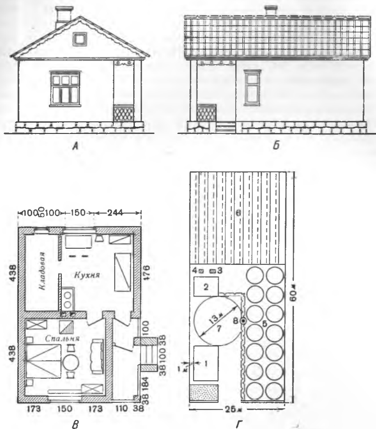
Рис. 4. План и внешний вид дома в селе Вилко. Постройка 1948 г. А — главный фасад, Б — боковой фасад, В — план жилища, Г — план усадьбы: 1 — жилой дом 53,9 м 2 , 2 — сарай 35 м 2 , 3 — уборная 1 м 2 , 4 — мусорный ящик 1 м 2 , 5 — сад 450 м 2 , 6 — огород 612,1 м 2 , 7 — хоз. двор 341 м 2 , 8 — колодец 1 м 2 ; общая площадь 1:00 м 2
