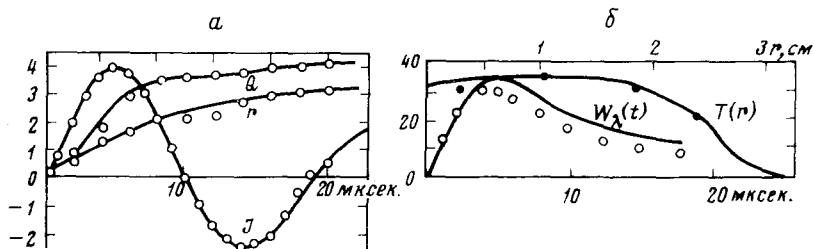
Рис. 3. Сравнение данных расчета и эксперимента (линия — расчет, точки — эксперимент). a : I — ток в 40 кА, r — граница интенсивного свечения в см, Q — выделение джоулева тепла по отношению к энергии батареи конденсаторов в 10%; б : Температура в 5 \cdot 10^{-2} эв на момент t=10 мксек. W_\lambda(t) — яркость по отношению к эталонному источнику в % на длине волны \lambda=5510 Å
