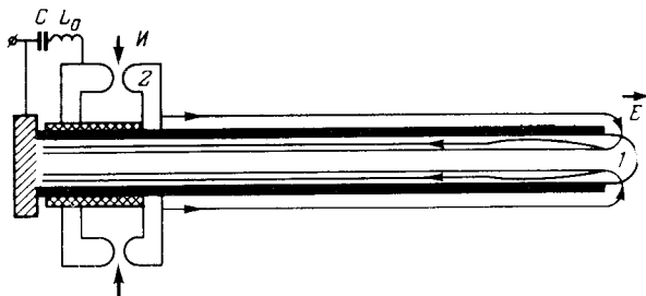
Рис. 1. Схема экспериментальной установки. C — емкость, L_0 — паразитная индуктивность, И — искровой разрядник; стрелки показывают направление тока, текущего от электрода 2 по плазменному цилиндру к электроду 1 — металлическому стержню, покрытому диэлектрической пленкой
