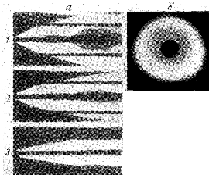
Рис. 2. Фотографии разрядов в ксеноне. a — фоторазвертки (СФР-граммы) для разрядов с начальным давлением 37 тор (1), 112 (2) и 600 тор (3); б — снимок разряда с торца, p=112 тор
